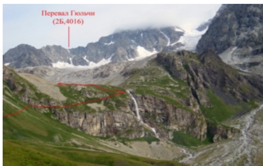
Фото № 166. Путь прохода из лощины к водопаду на реке Орс-дон.
