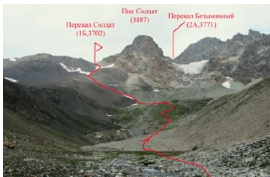
Фото № 180. Путь подхода к перевалу Солдат с востока.
