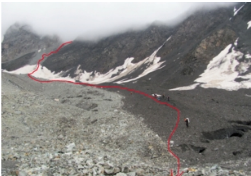
Фото № 188. Спуск с перевала Солдат по леднику Безымянный.
