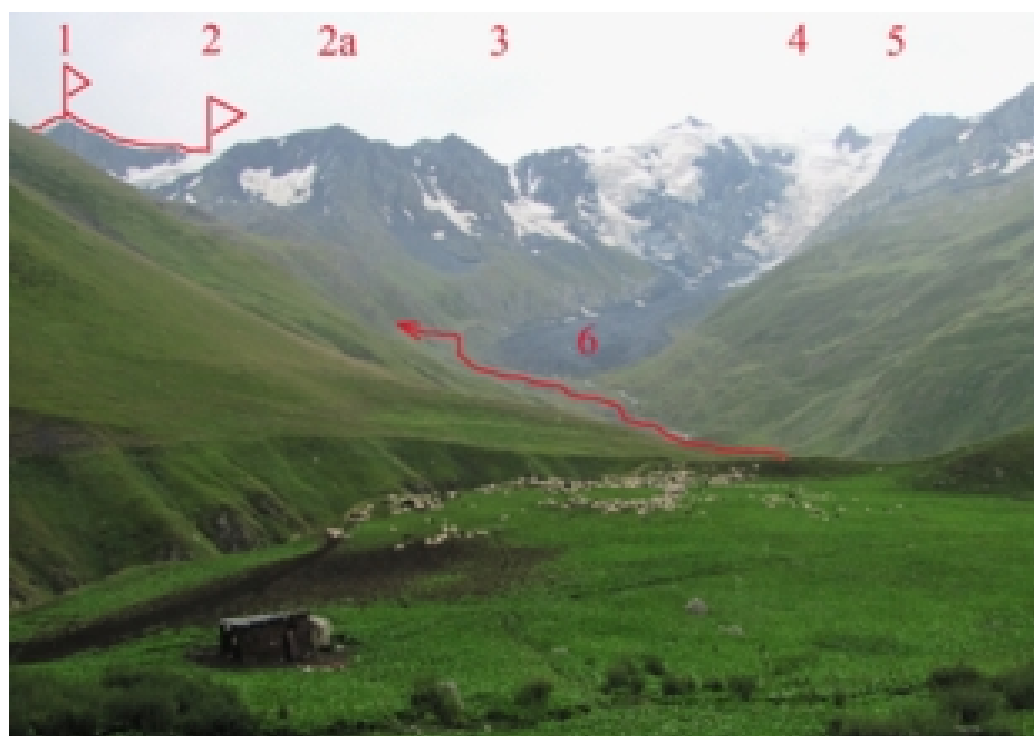
Фото № 192. Вид на истоки реки Карасу: 1 – пик Штулу-Тау (3597), 2 – перевал Джераска (2А,3470), 2а – пик Джераскифастакалхойне (3562), 3 – перевал Гуцулочка (2А,3411), 4 – пик Гезе-Тау (4009), 5 – перевал Эдена, 6 – ледник Штулу восточный.
