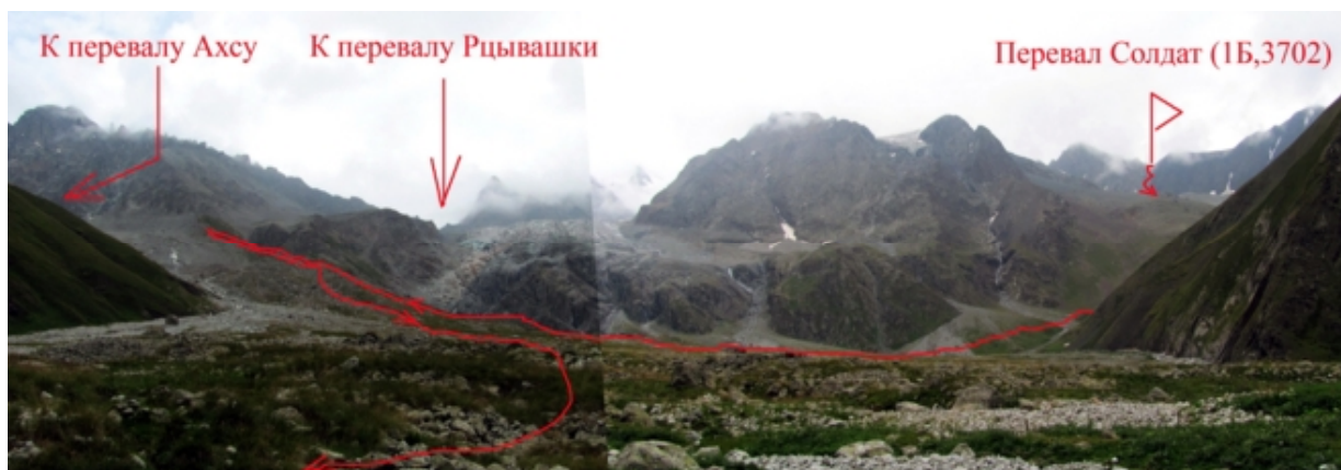
Фото № 191. Верховья реки Ахсу. Место ухода на запасной вариант.
