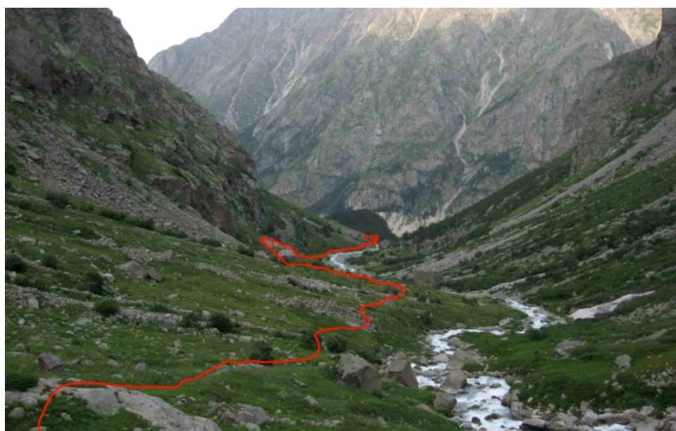
Фото № 254. Вид на долину реки Фастаг от устьевой ступени ущелья Харески.
