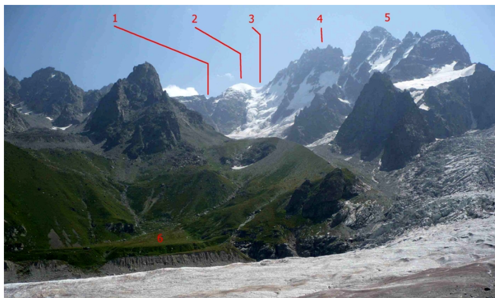
Фото № 268. Вид с левобережной морены ледника Караугом на восток: 1 – перевал Воологата (2Б,4000); 2 – Купол Воологаты (4150); 3 – перевал Караугом-Гулар (3А,4000); 4 – пик Караугом-хох восточный (4520); 5 – пик Караугом-хох западный; 6 – поляна Микелай.
