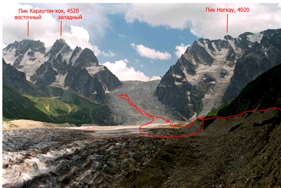
Фото № 265. Ледник и ледопад Караугом.
