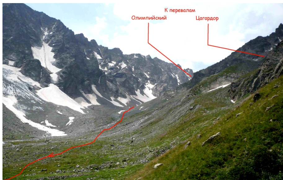
Фото № 252. Устьевая ступень ущелья Цагардор восточный.
