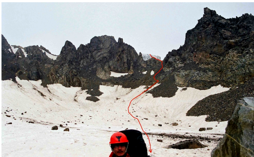
Фото № 247. Восточный цирк перевала Олимпийский (2Б,4060) с ледника Фастаг.
