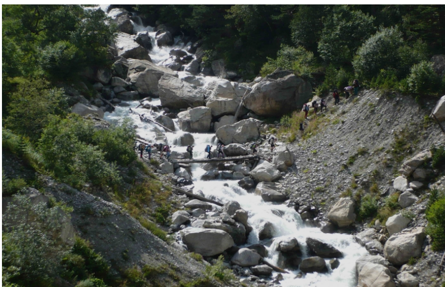
Фото № 263. Мост через реку Фастаг-дон.
